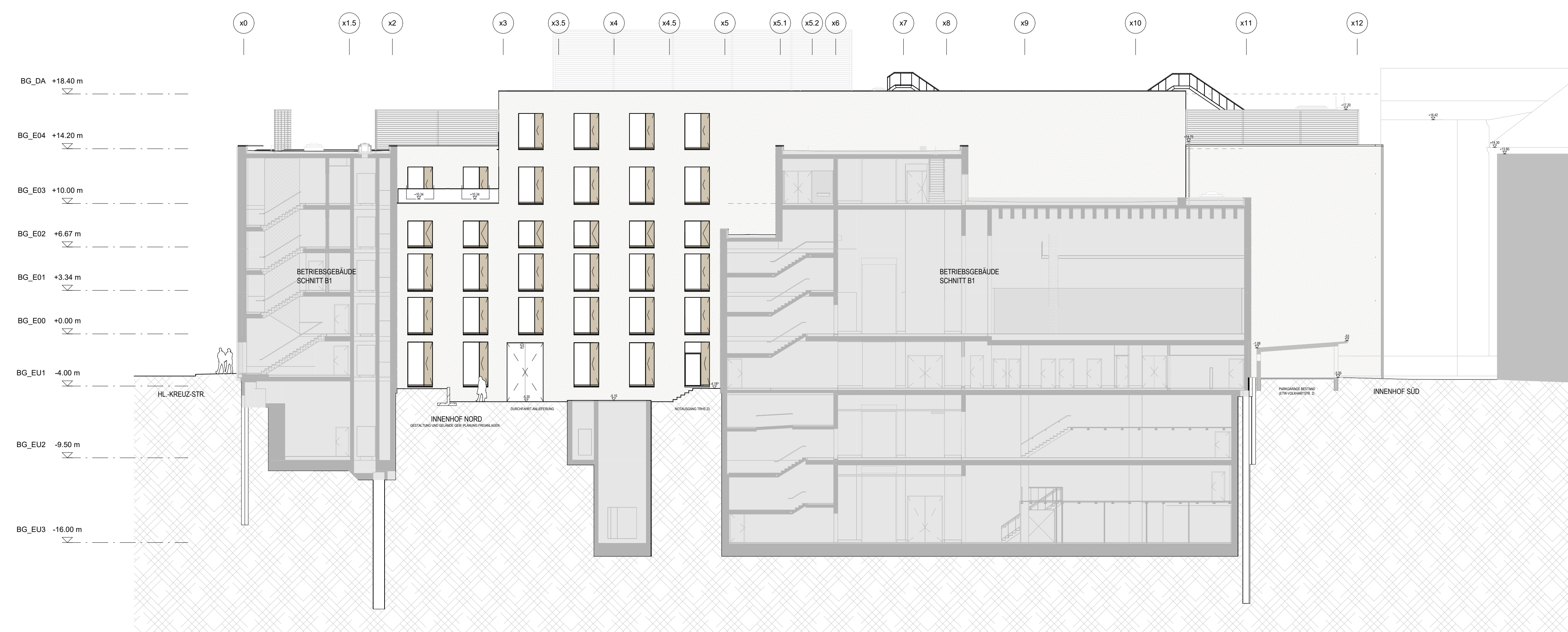
Ansicht 04a - Innenhof Nord 1 : 200
