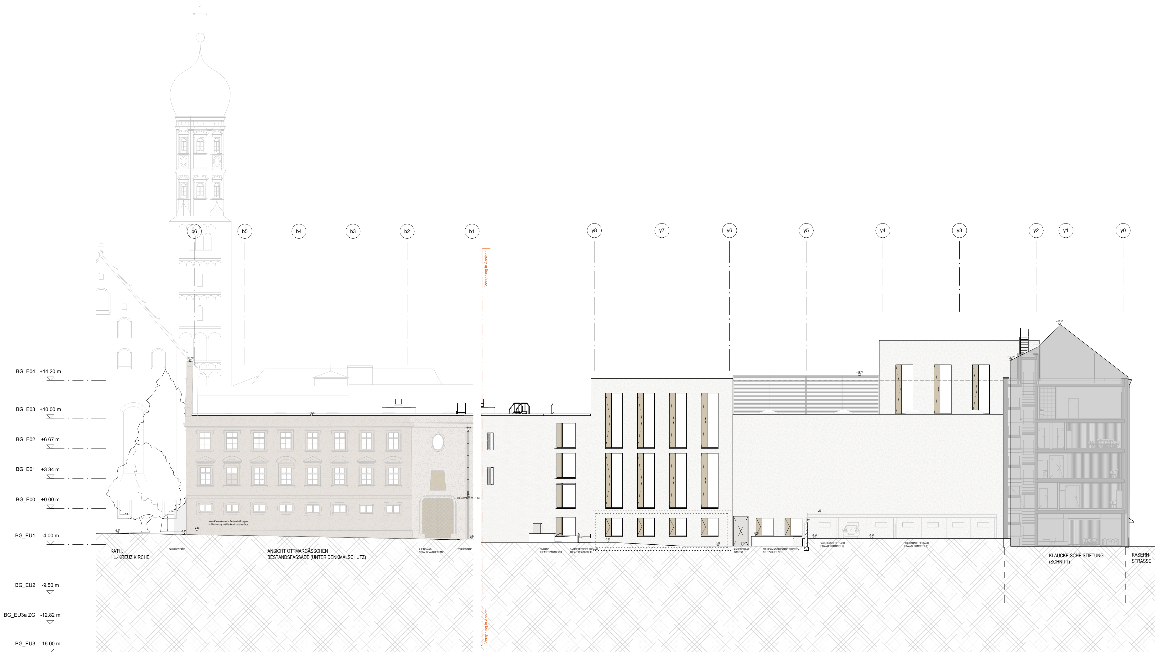
Ansicht 03 - Volkmarstraße, Ottmargälschen 1 : 200
